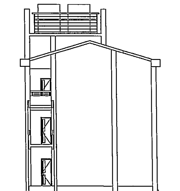
0. FACADE LATÉRALE DROITE 1:125
